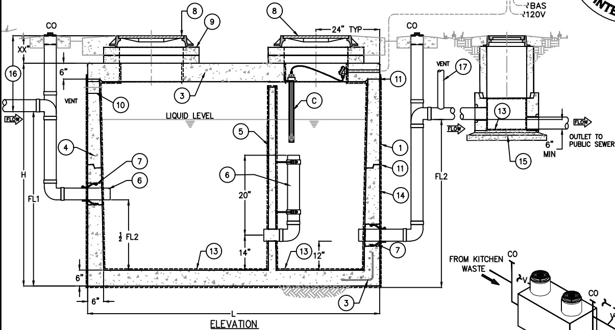
ELEVATION
